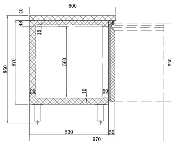
ABBILDUNG ZEIGT VERSION OHNE AUFKANTUNG
